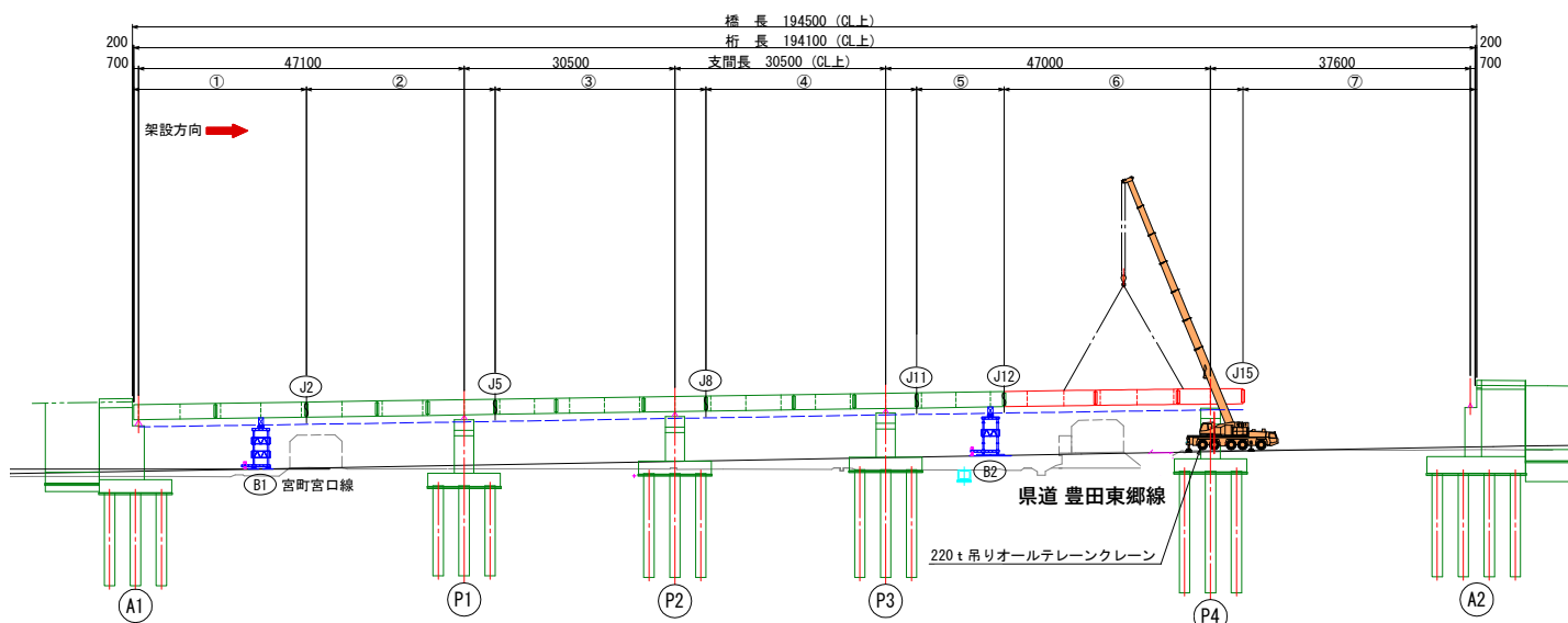
側面図
