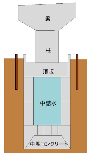
STEP④ 躯体施工
