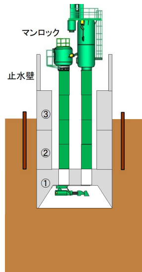
STEP③ ニューマチック ケーソン基礎施工②
