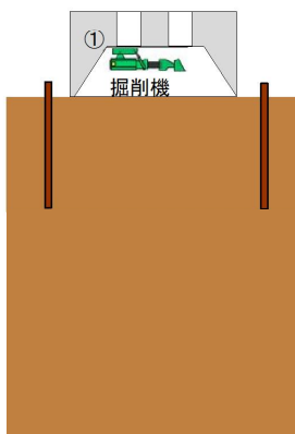
STEP② ニューマチック ケーソン基礎施工①
