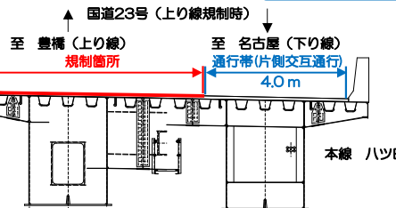
規制箇所 横断図（A-A'）
