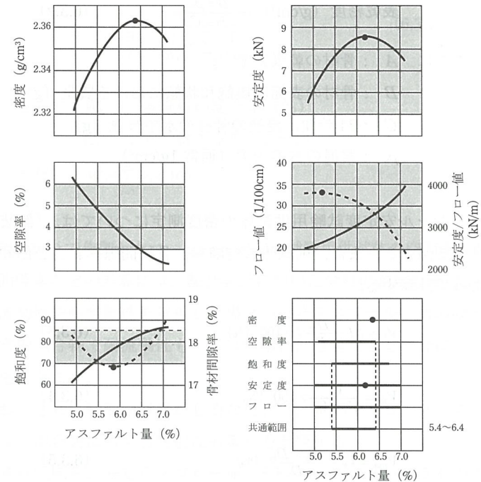
図-6.3.3 設計アスファルト量の設定
