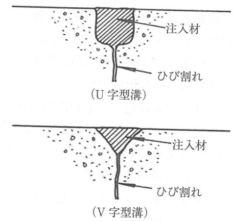
図-4.2.5 コンクリート舗装における進行性ひび割れのシール溝形状
