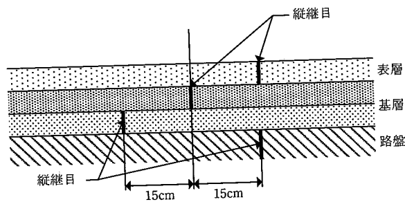
図-6.4.2 各層縦継目の一例
