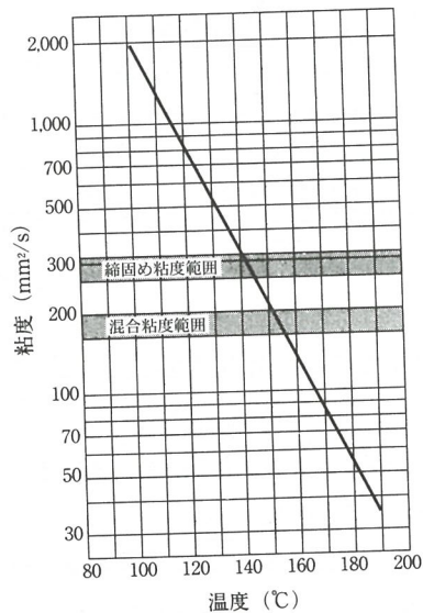
図-6.3.2 アスファルトの温度粘度関係の一例
