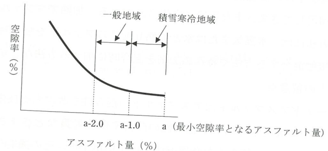
図-9.4.2 アスファルト量の選定範囲の例
