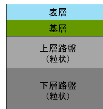
(一般的なアスファルト舗装の構成)
