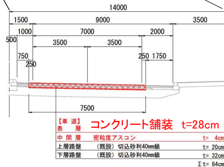
標準定規図
