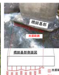
橋脚の洗掘
