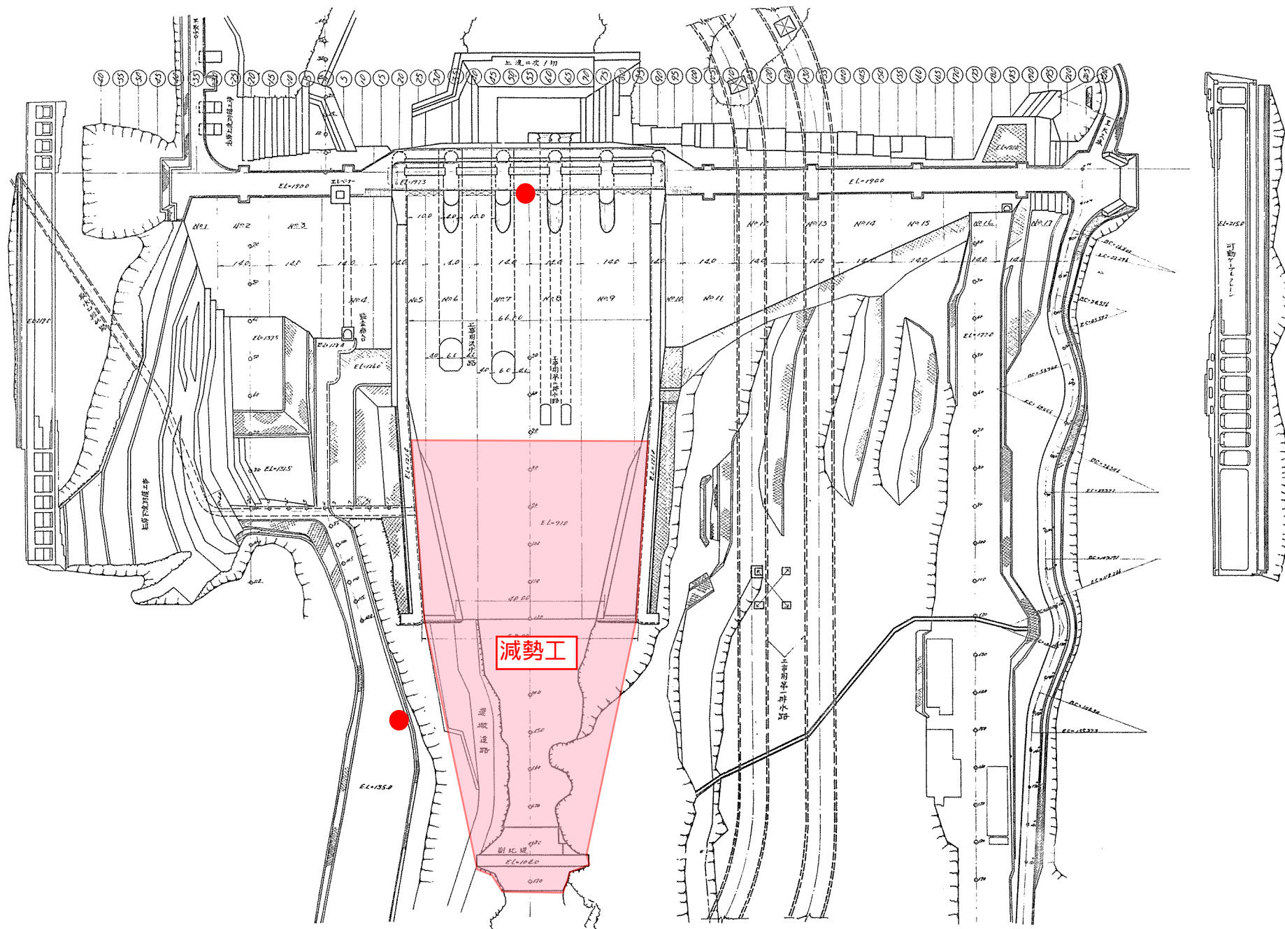
附圖(土) — 6 ダム平面図
