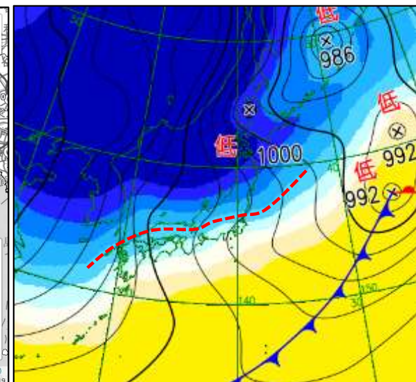
上空850hPa (約1500m付近)の気温 -18.0 -15.0 -12.0 -9.0 -6.0 -3.0 0.0 3.0 °C --- 上空約1500mの気温-9°C (平地で大雪となる目安)
