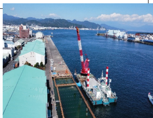
裏込・裏埋工
