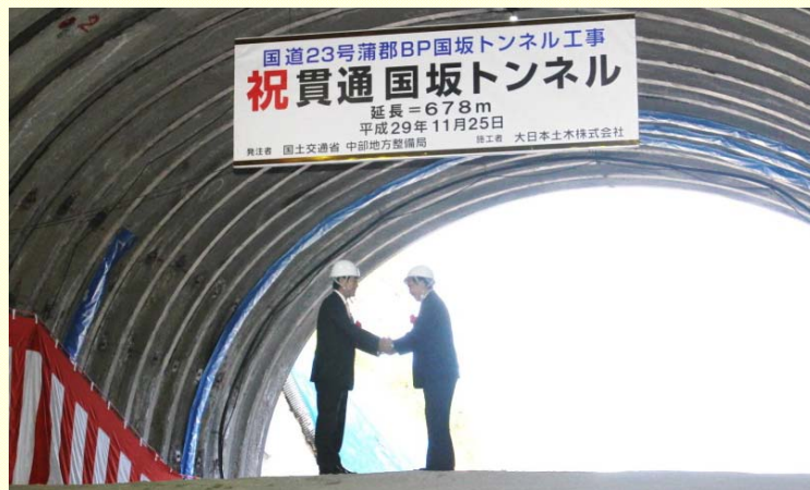
11月25日 国道23号蒲郡バイパス(名豊道路)国坂トンネル(仮称)貫通式 蒲郡市長と豊川市長による通り初めの様子 (名四国道事務所)
