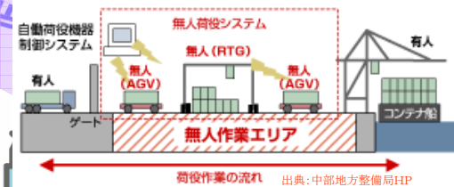
コンテナターミナルの自動化荷役 (イメージ図)
