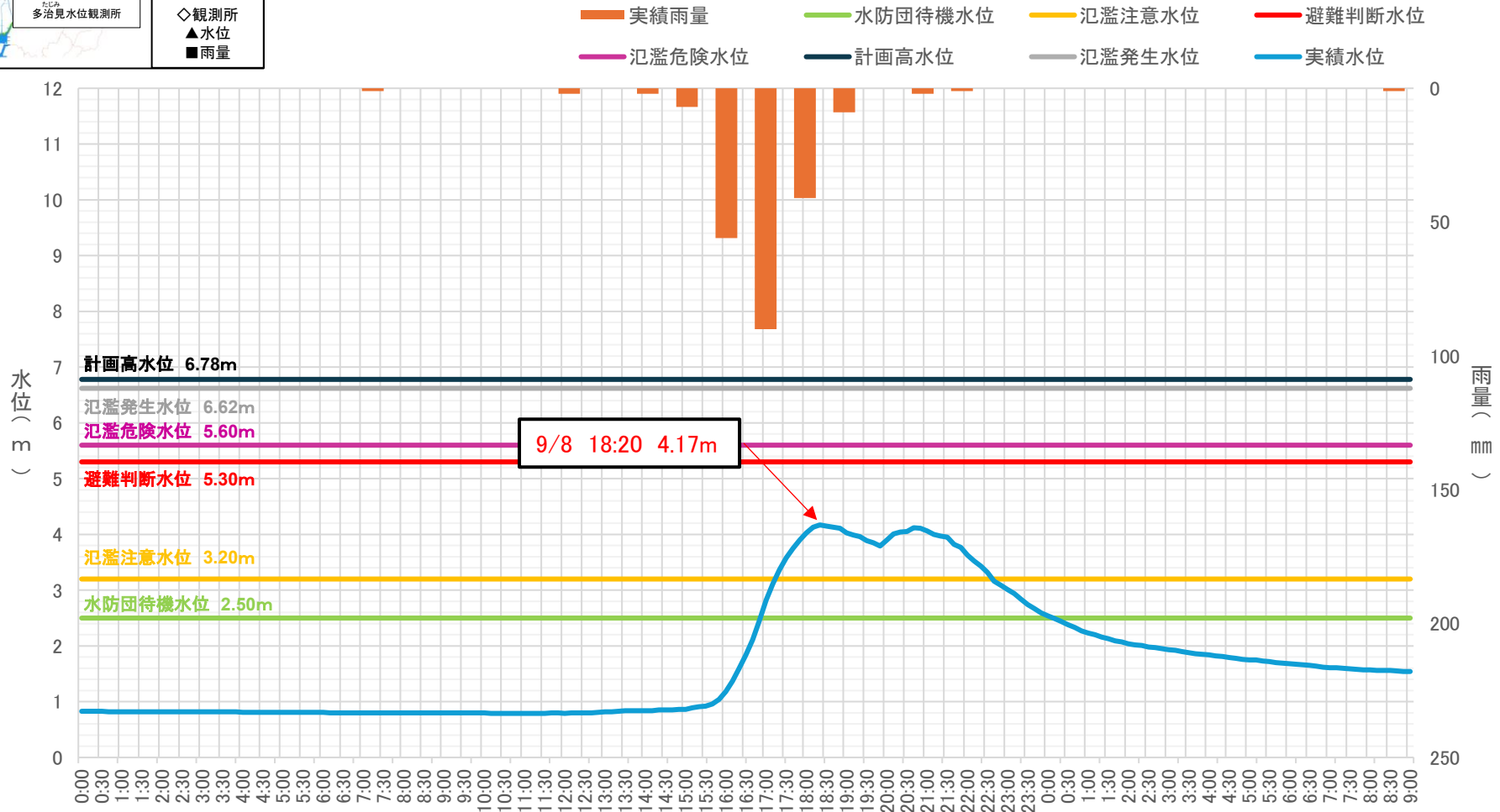
たじみ 多治見水位観測所の実績水位と多治見雨量観測所の実績雨量
