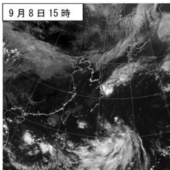
9月8日15時 気象衛星赤外画像
