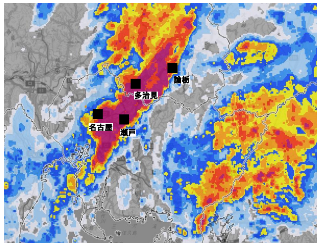
9月8日16時50分 レーダー雨量 出典：気象庁WEBページ
