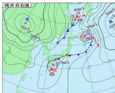
9月8日15時 地上天気図
