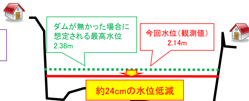
B'-B 市原水位観測所 (国道19号小里川橋付近)の模式断面図
