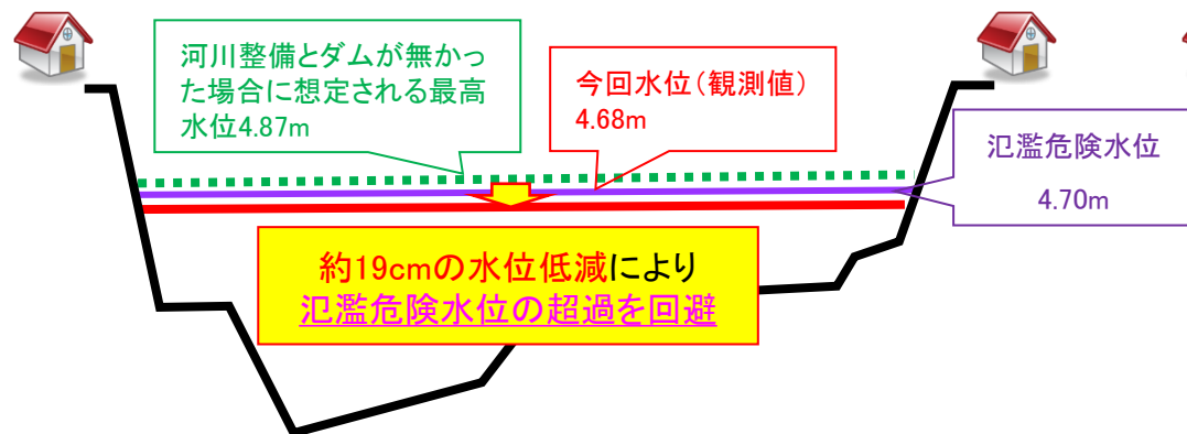
A'-A 土岐水位観測所 (河口から57.8k付近)の模式断面図
