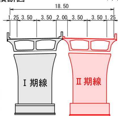
標準横断面図 (単位:m)
