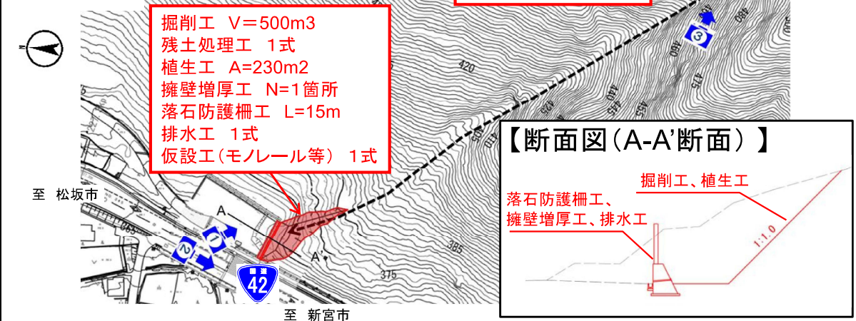
【平面図】
