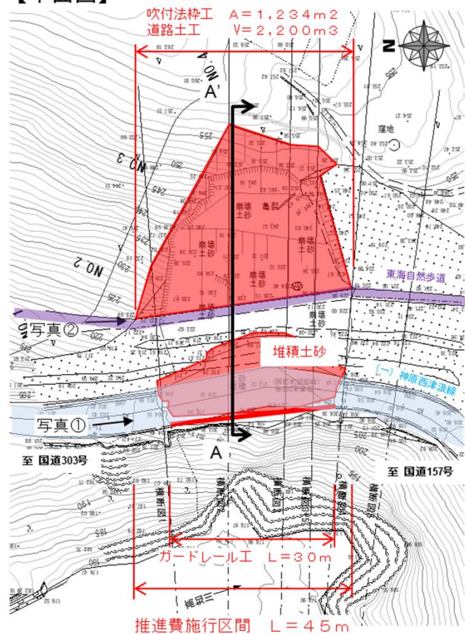
【平面図】
