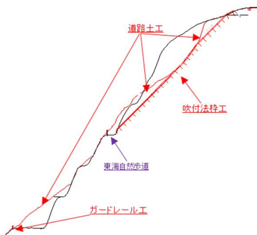
【断面図(A-A')】
