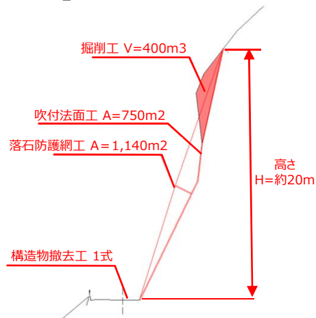
【断面図】A-A'断面
