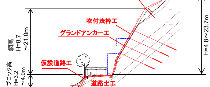
【断面図】A-A'断面
