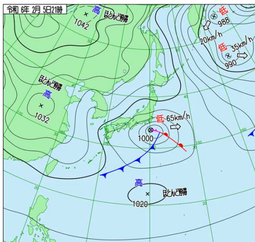
天気図(2月5日21時)
