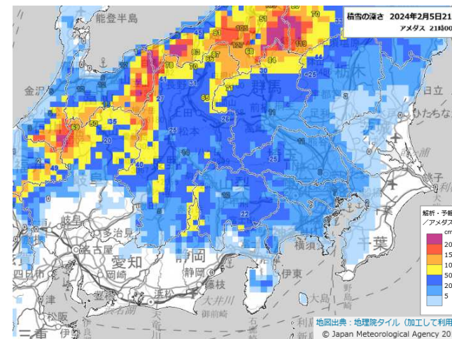
解析積雪深(2月5日21時)
