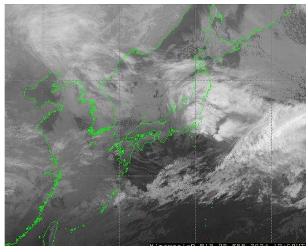
気象衛星赤外画像(2月5日21時)
