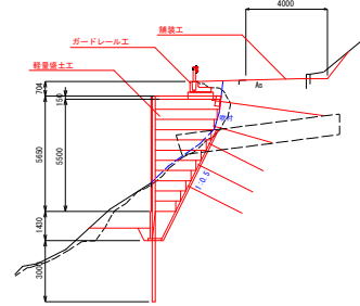
【断面図】A-A'断面
