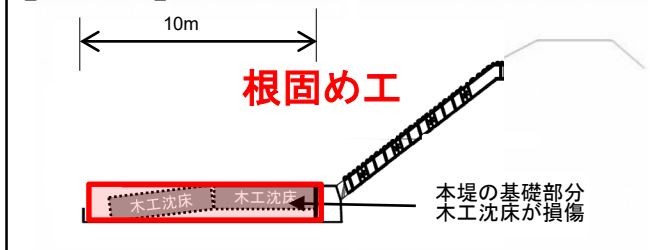
【断面図】 A-A' 断面
