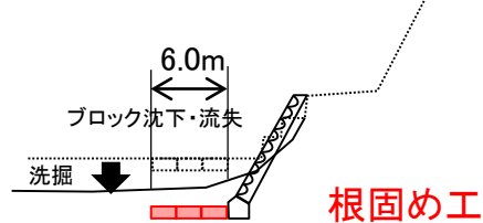
【断面図】 A-A' 断面
