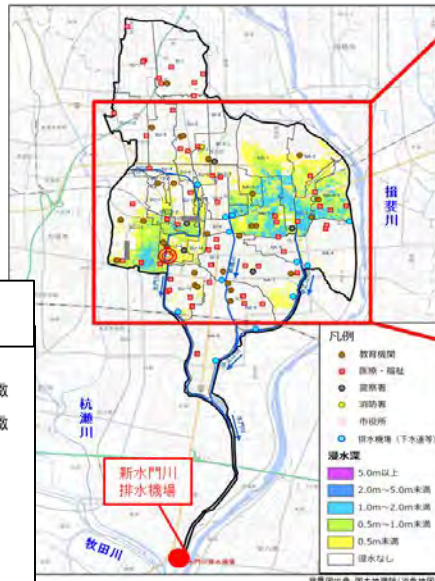
昭和36年6月洪水と同規模の洪水が発生した場合に想定される浸水区域及び重要施設位置
