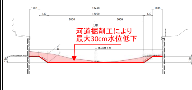
【横断図(7K700)】
