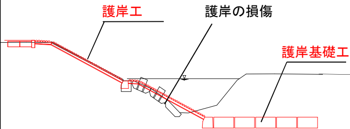
【断面図A-A'】
