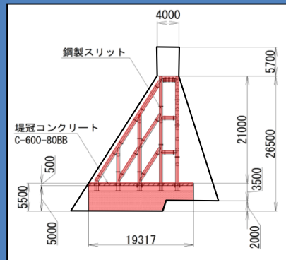
横断面図
