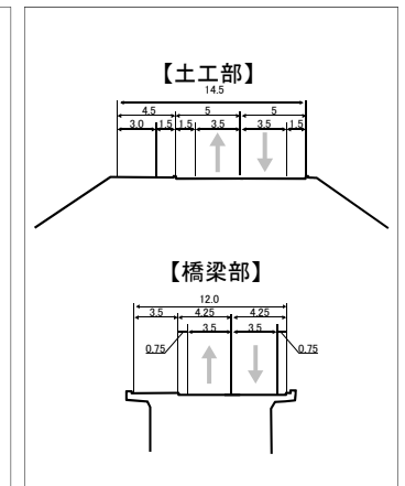
【横断面図】
