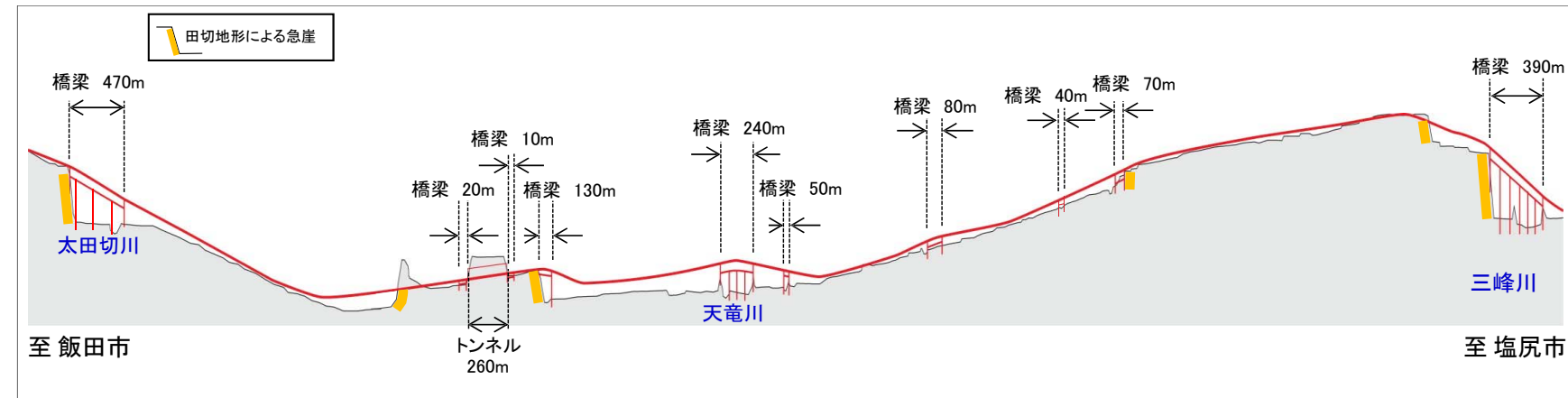
【縦断面図】
