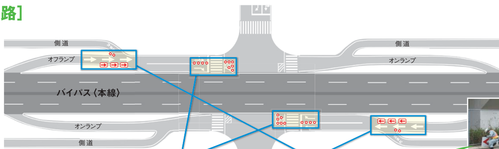
ラバーポール・矢印路面表示・高速出口路面表示・進入禁止看板を設置
