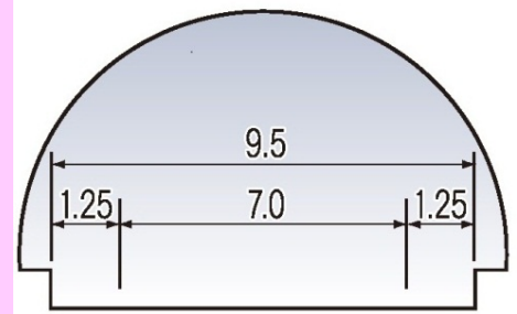
トンネルの完成断面
