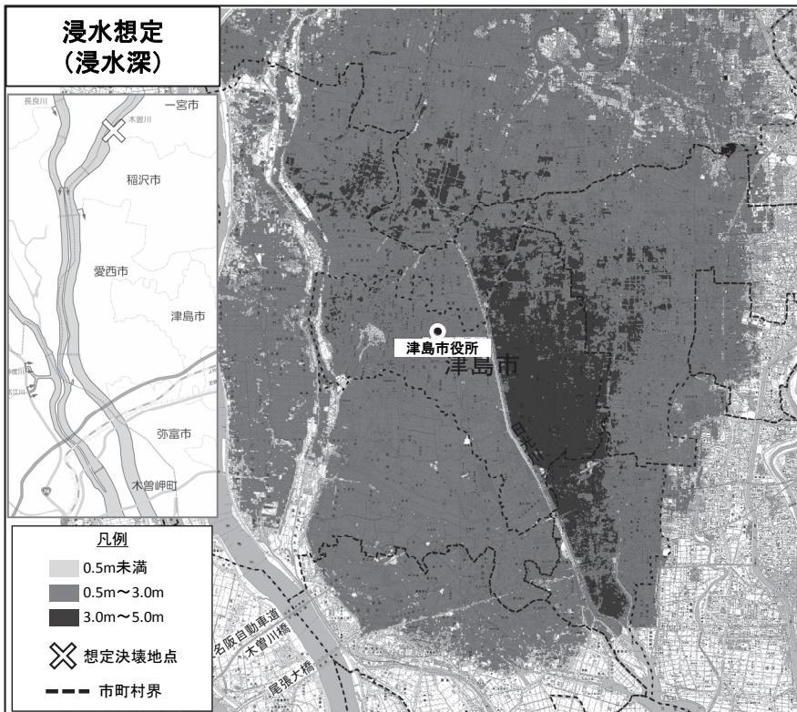
木曾川左岸29.2km地点決壊(29時間後)
