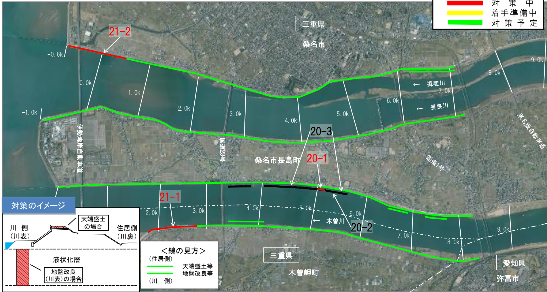
図：河川整備計画における工事实施(予定)箇所図
