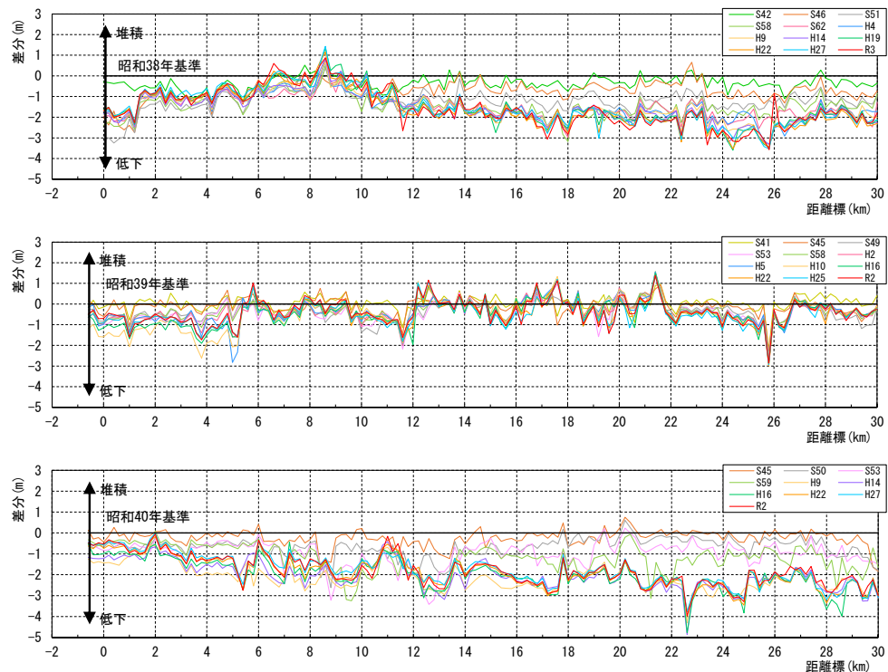
図 2-4 平均河床高の過去の低下状況と近年の安定
