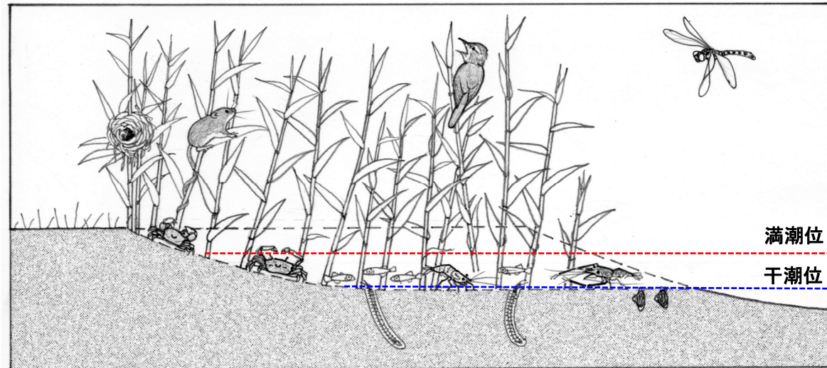
図 5-3 ヨシ原の再生イメージ（高水敷切下げ）
