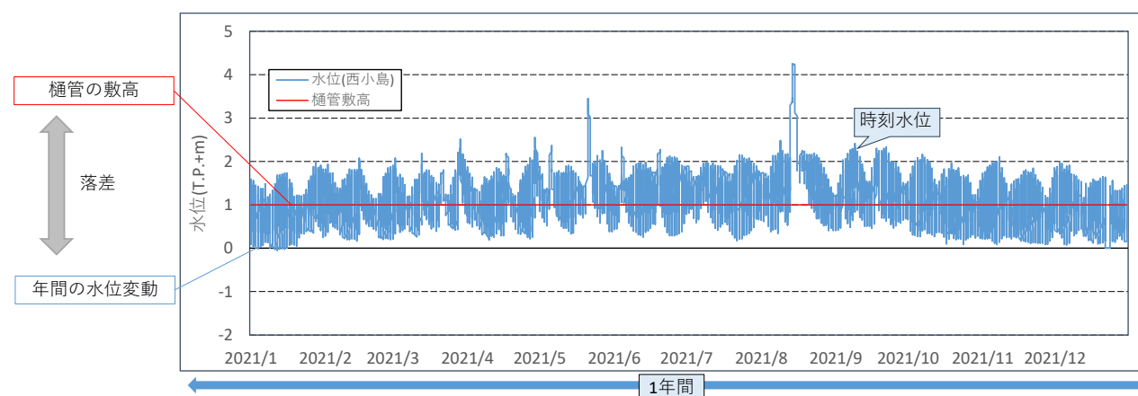
図 3-8 時刻水位の年変動と樋管の敷高の関係（揖斐川 22k 上野河戸排水樋管）
