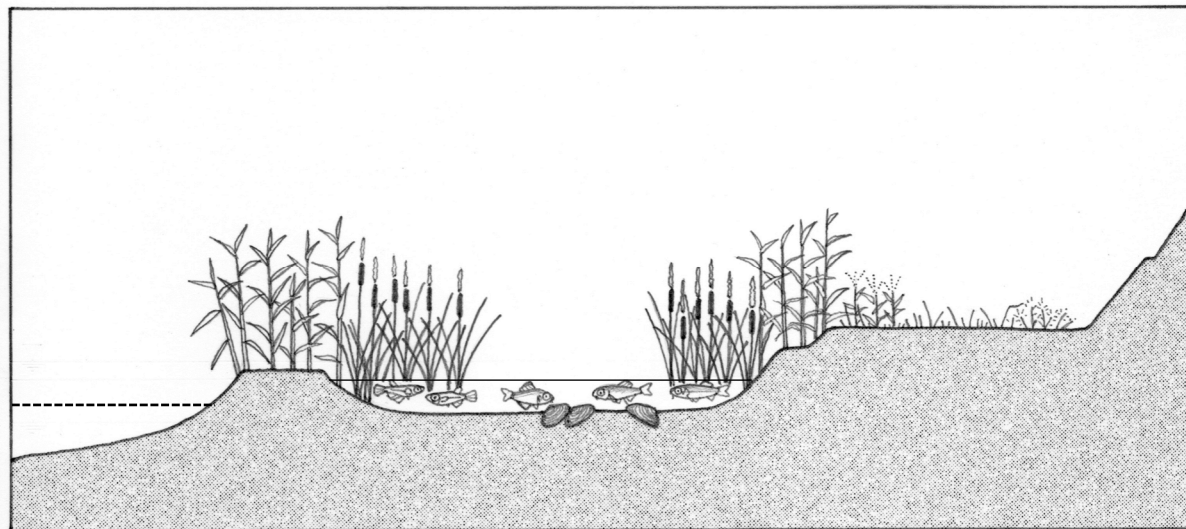
図 5-1 上流におけるワンド等の再生イメージ（地盤切り下げ）
