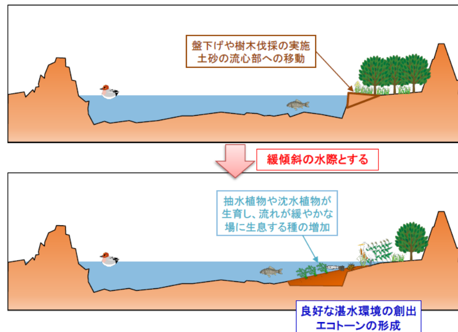
図 5-4 良好な湛水環境の整備イメージ（横断図）
