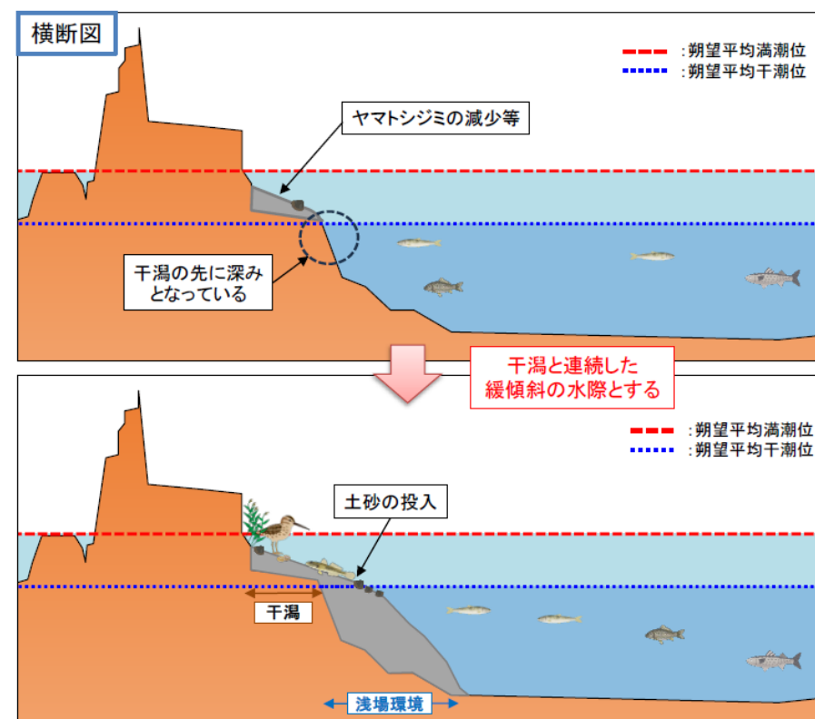
図 5-7 浅場環境の整備イメージ（横断面図）
