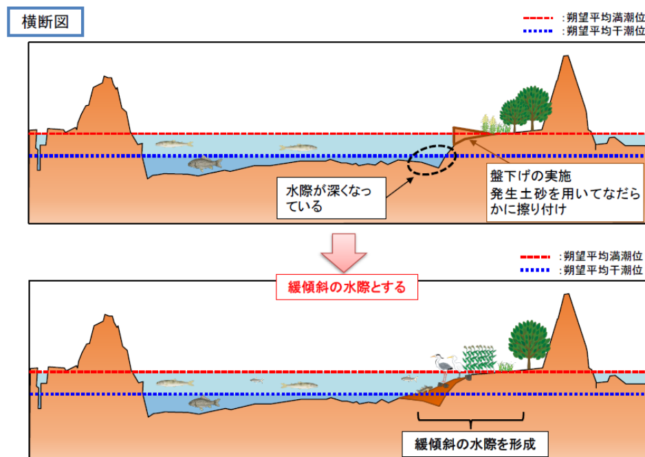
図 5-9 浅場環境の整備イメージ（横断面図）
