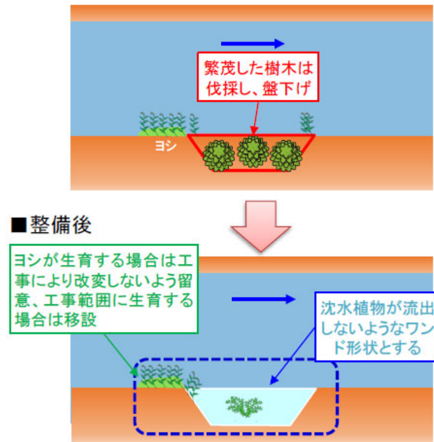
図 5-5 良好な湛水環境の整備イメージ（平面図）
