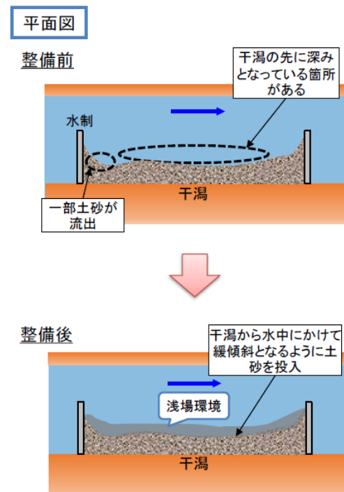
図 5-8 浅場環境の整備イメージ（平面図）
