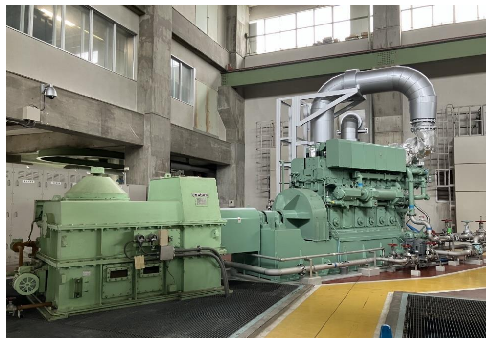
1号主原動機完成
