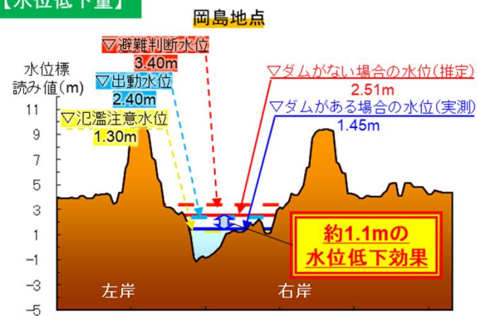
【水位低下量】
