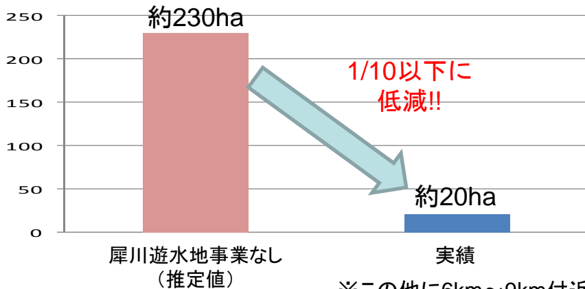
犀川遊水地事業による浸水面積低減効果(犀川5km付近)
