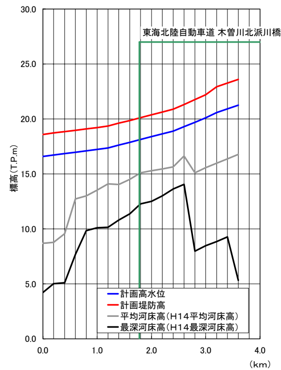
計画諸元表・北派川
