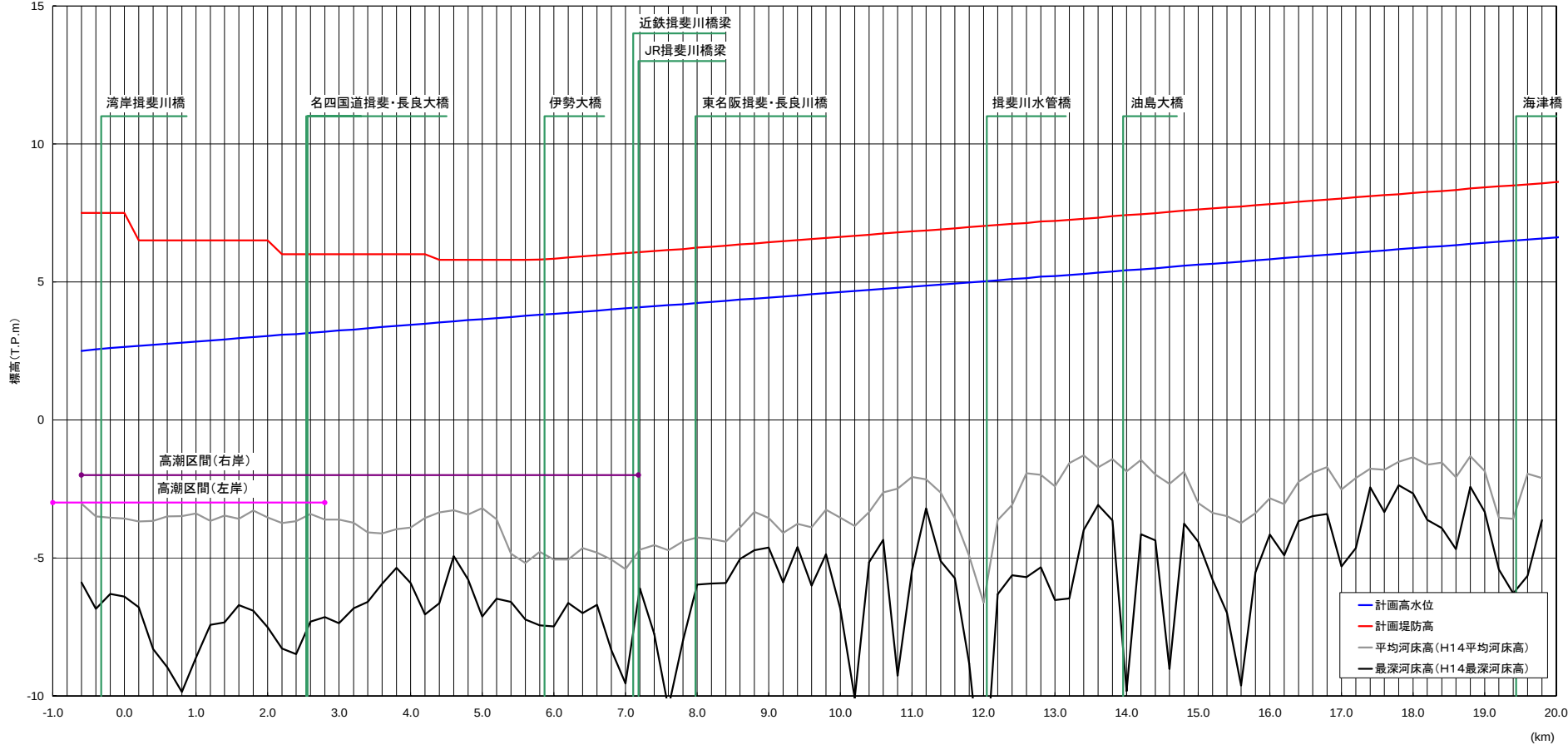
計画諸元表・揖斐川(0.0k~19.8k)
