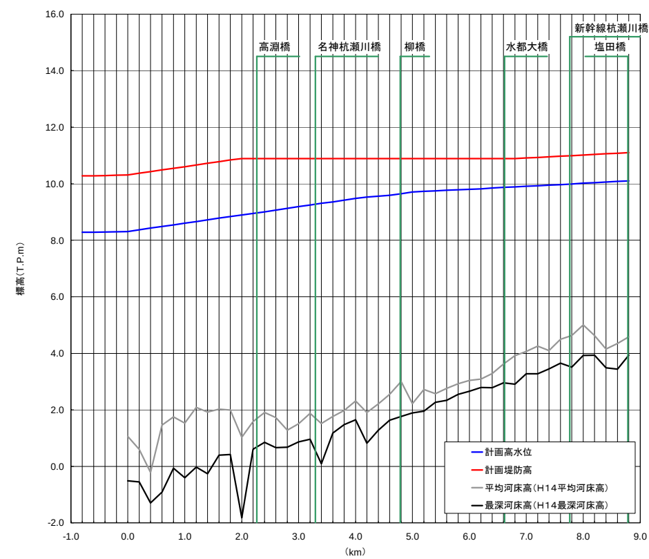
計画諸元表・杭瀬川
