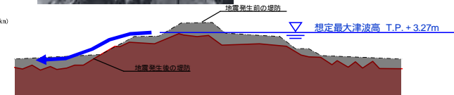
地震による堤防の沈下（木曽川左岸4.0k(現況)）
