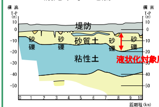
木曽川（左岸）土質縦断面 (0~10km)
