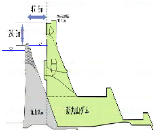
■ダム標準断面図
