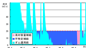
摂斐川万石地点の流況
