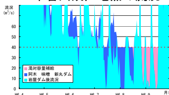
木曽川成戸地点の流況
