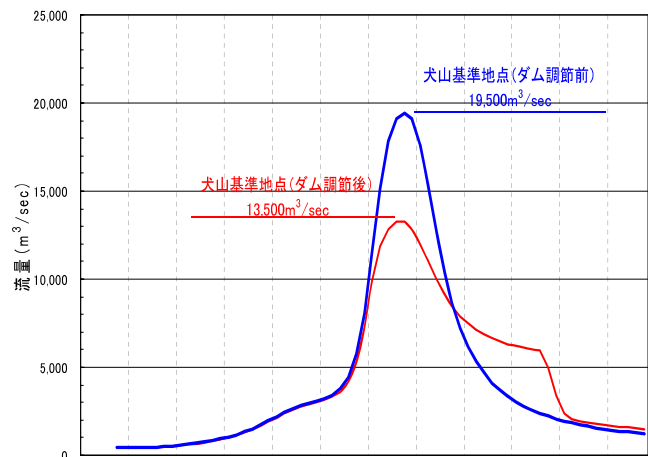
犬山基準地点（昭和58年9月洪水型）
