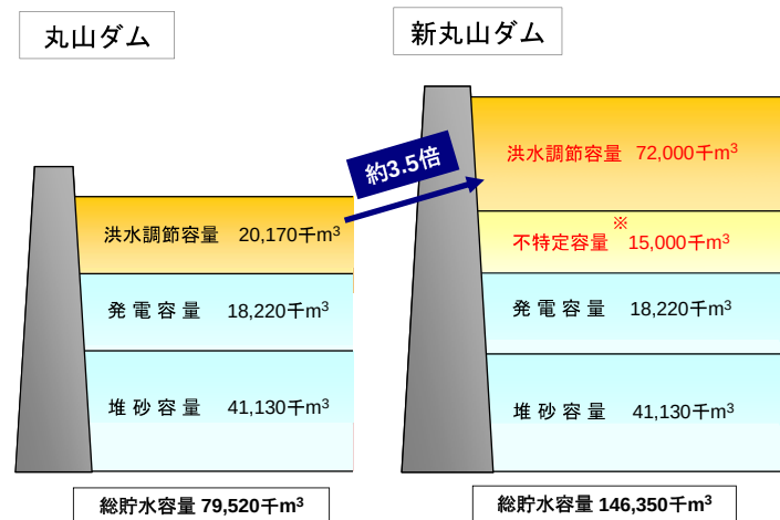
■貯水容量配分図
