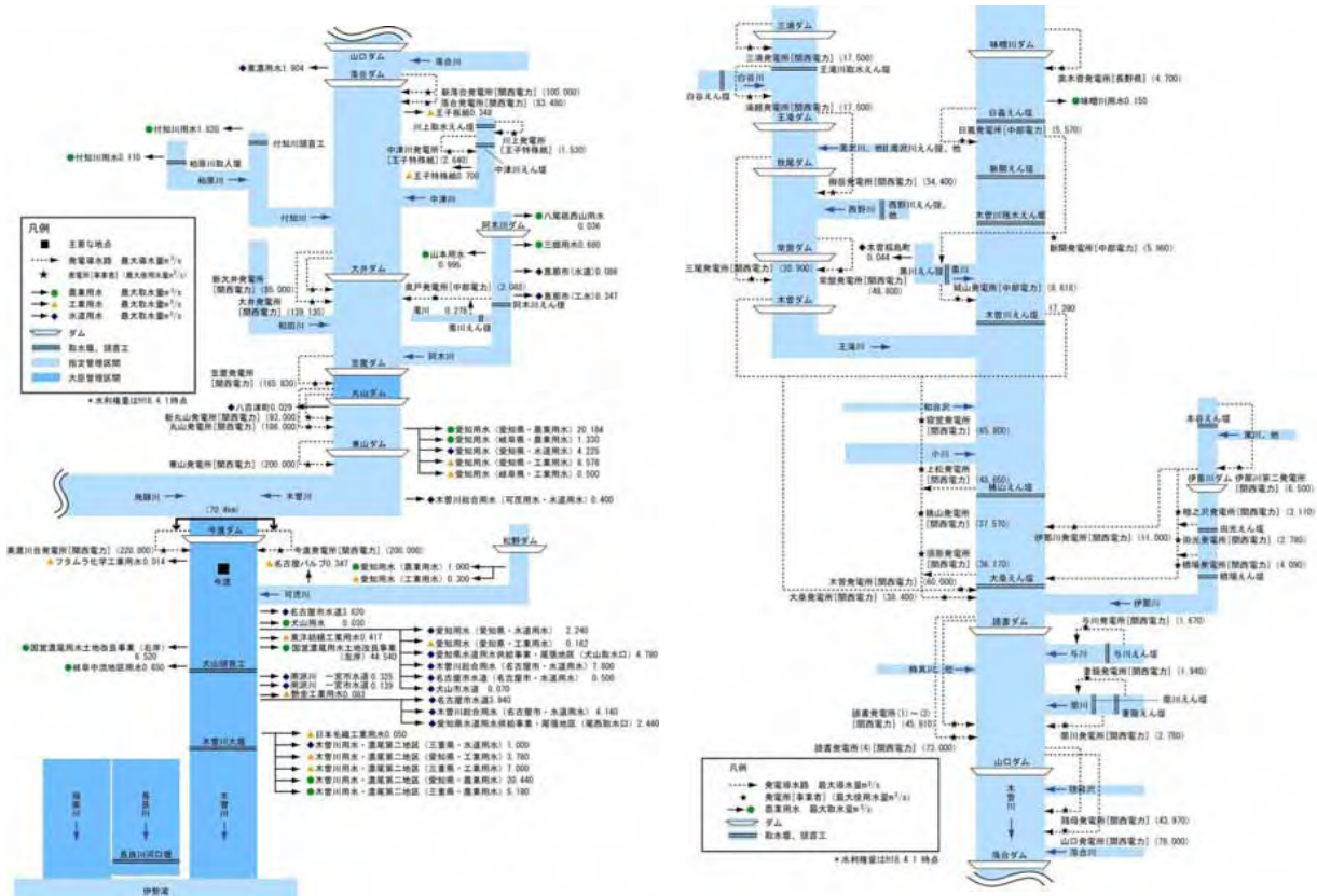
木曽川水利模式図(1/2)(主要な水利権を記載)
