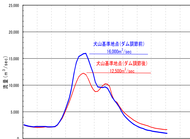
犬山基準地点（昭和35年8月洪水型）
