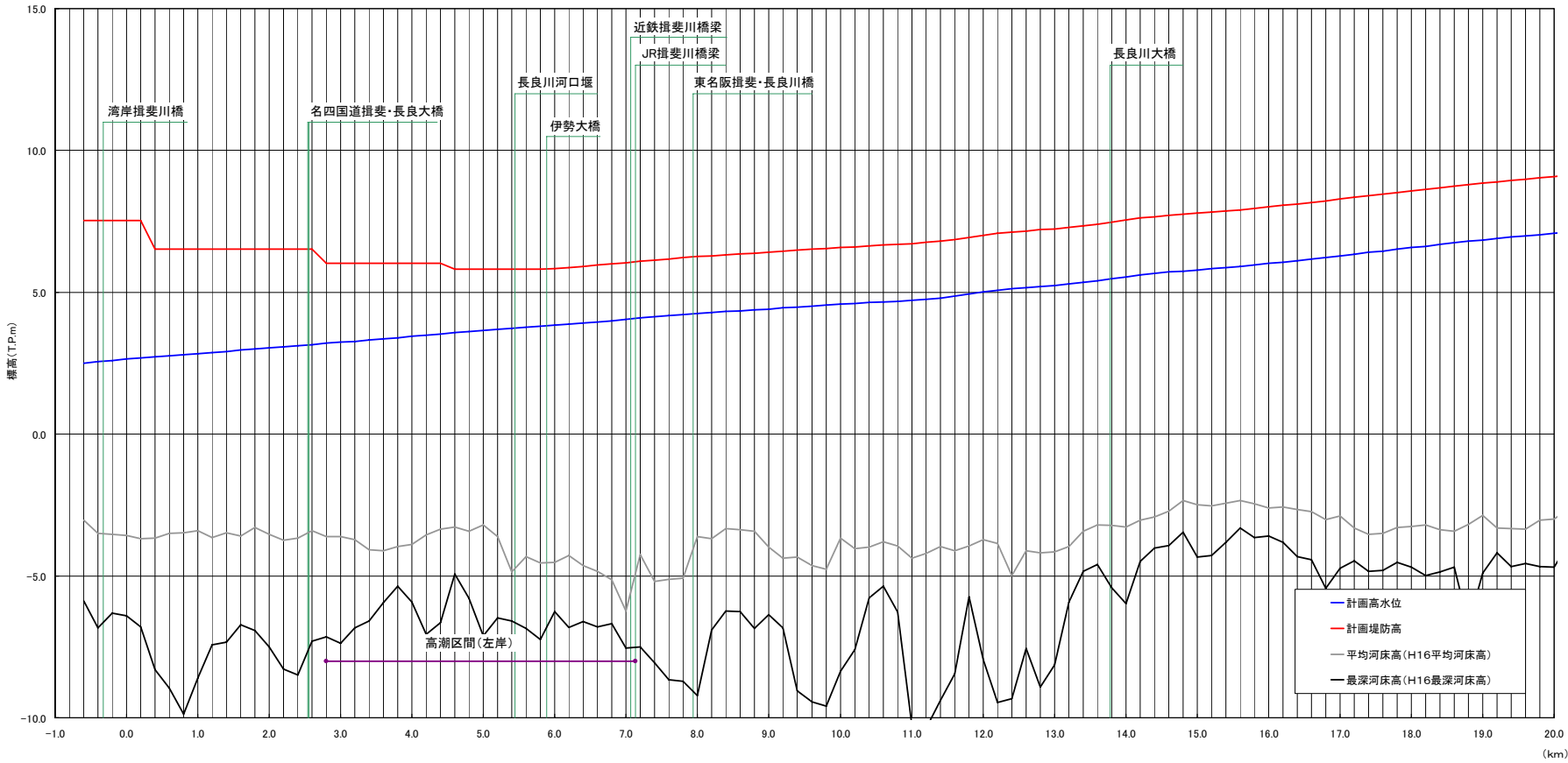
計画諸元表・長良川(-0.60k~19.8k)
