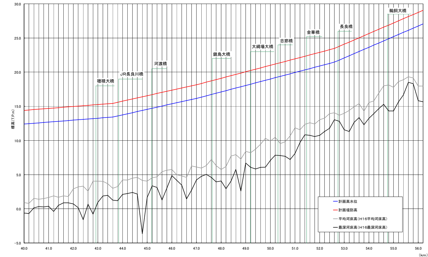
計画諸元表・長良川(40.0k~56.2k)
