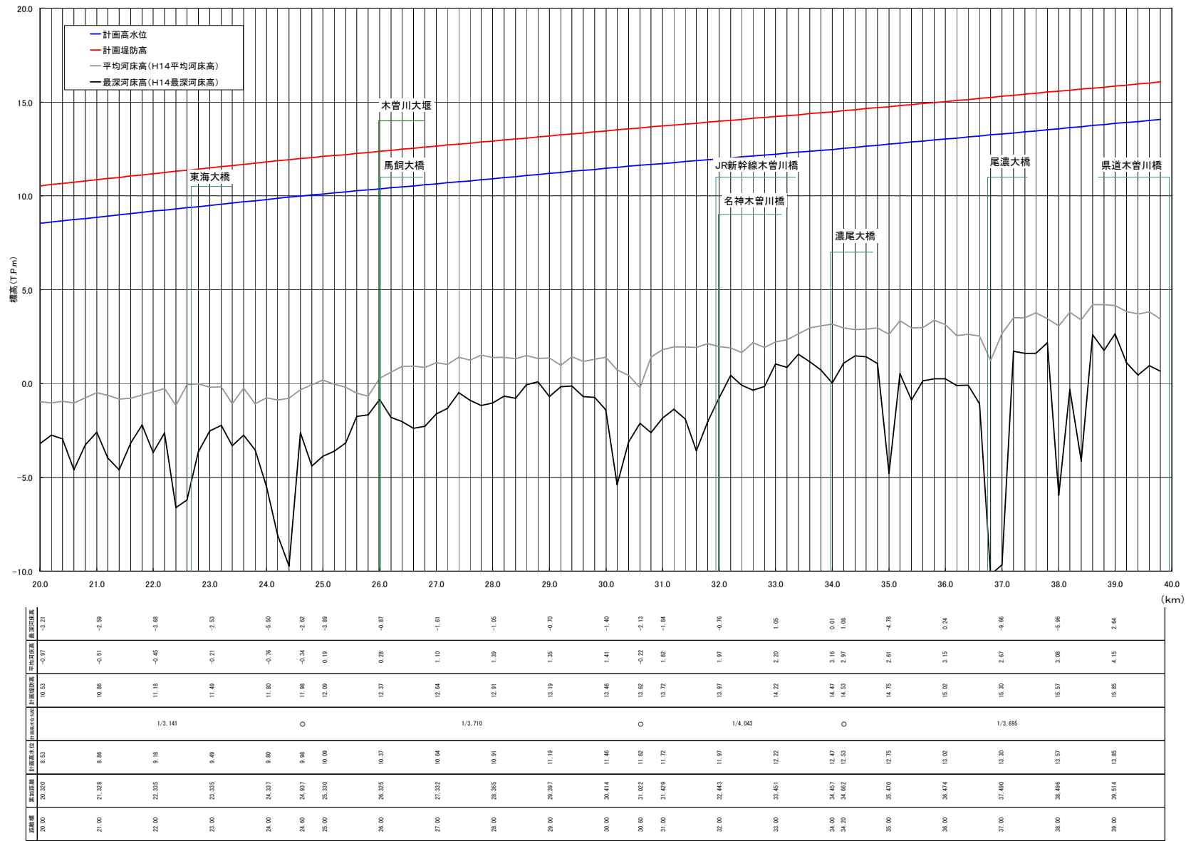
計画諸元表・木曽川(20.0k~39.8k)
