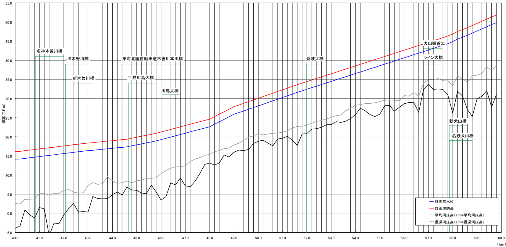
計画諸元表・木曽川(40.0k~59.8k)
