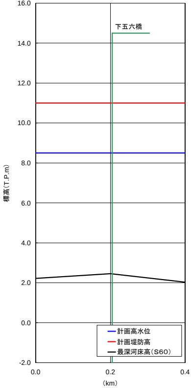
計画諸元表・五六川
