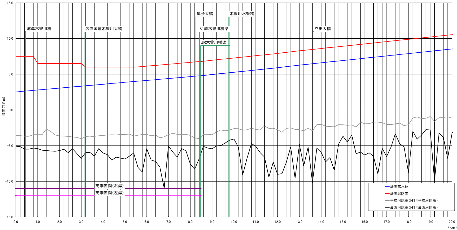
計画諸元表・木曽川(0.0k～19.8k)
