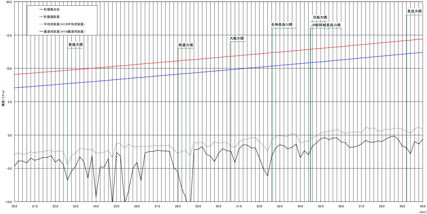
計画諸元表・長良川(20.0k~39.8k)
