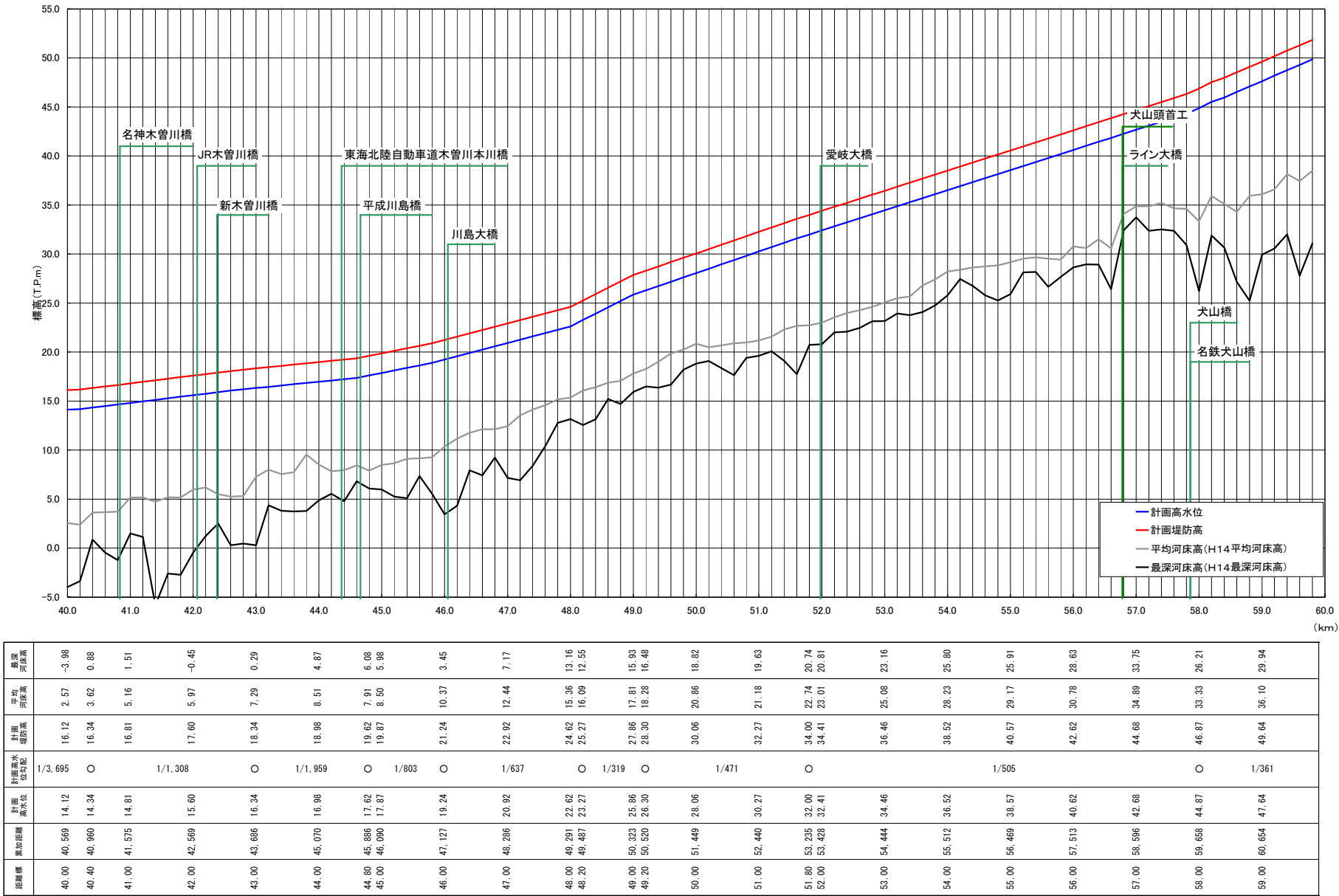
計画諸元表・木曽川(40.0k~59.8k)
