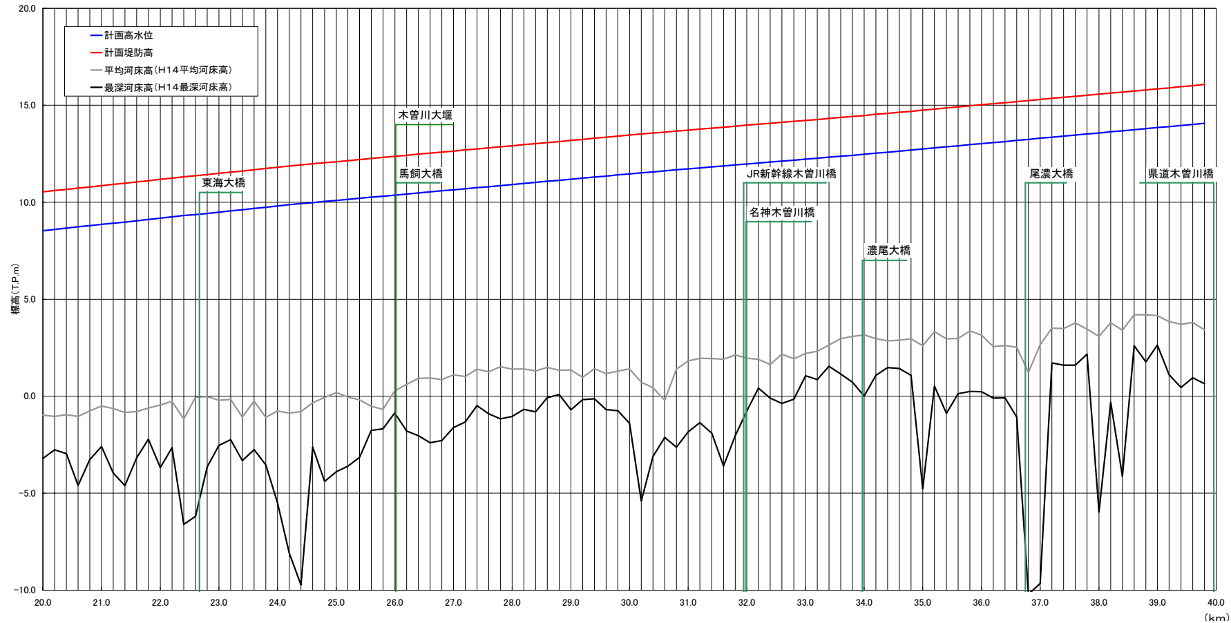
計画諸元表・木曽川(20.0k~39.8k)
