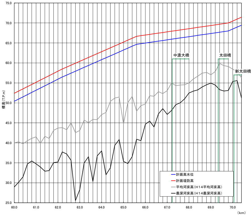
計画諸元表・木曽川(60.0k~70.4k)
