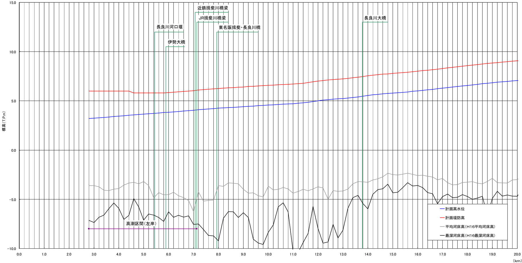
計画諸元表・長良川(2.8k~19.8k)
