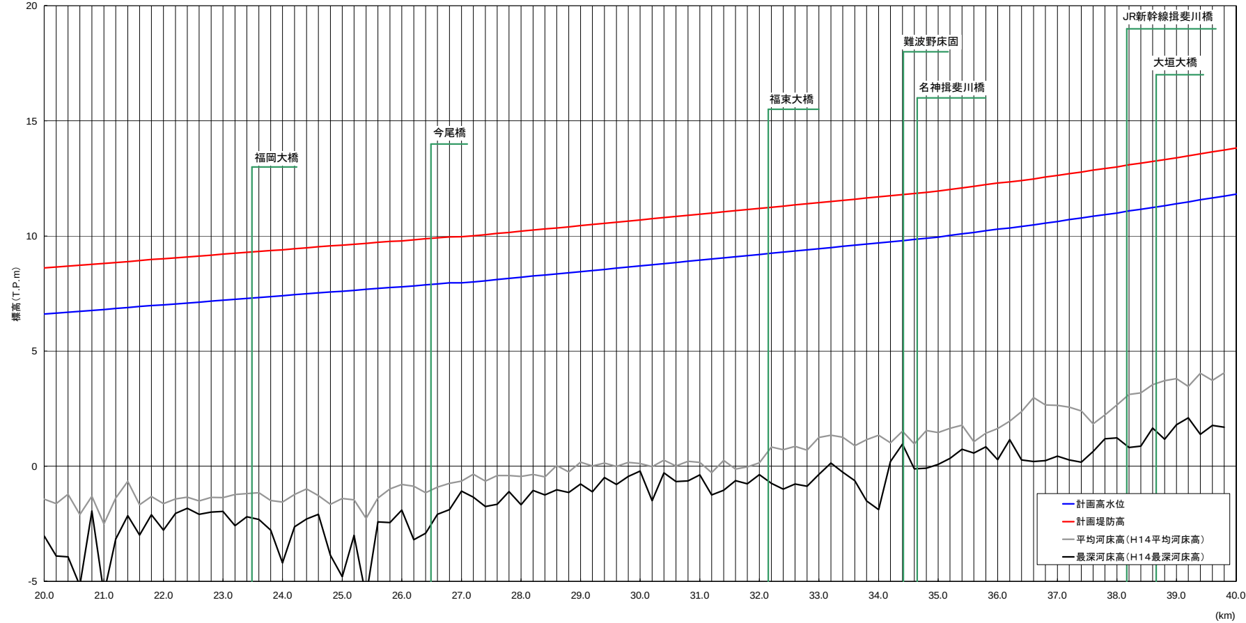
計画諸元表・揖斐川(20.0k~39.8k)
