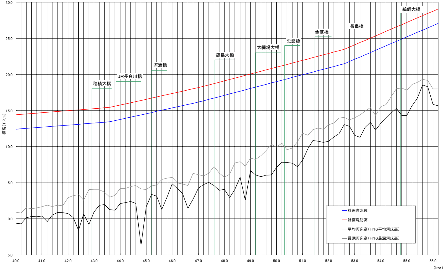
計画諸元表・長良川(40.0k~56.2k)
