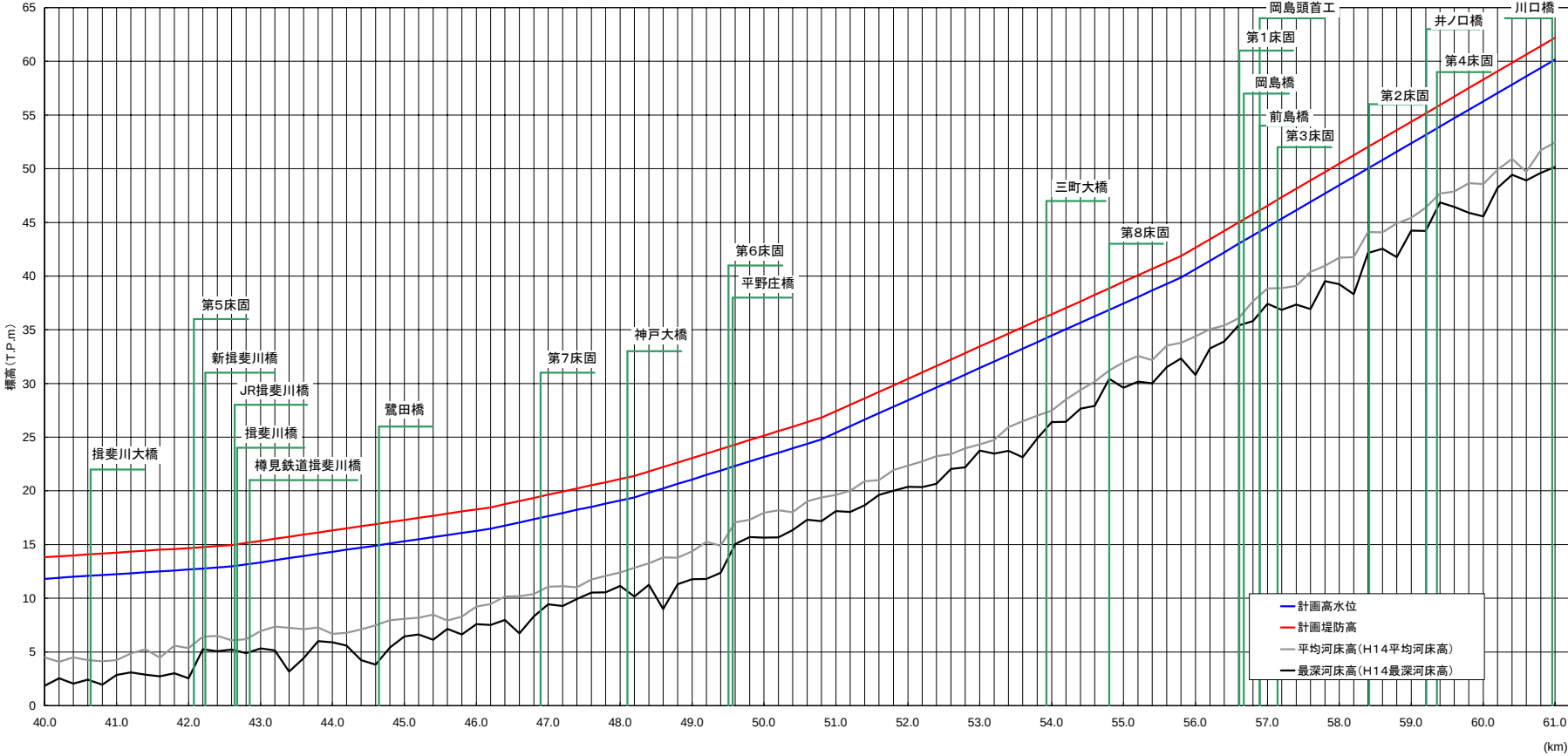
計画諸元表・揖斐川(40.0k~61.0k)
