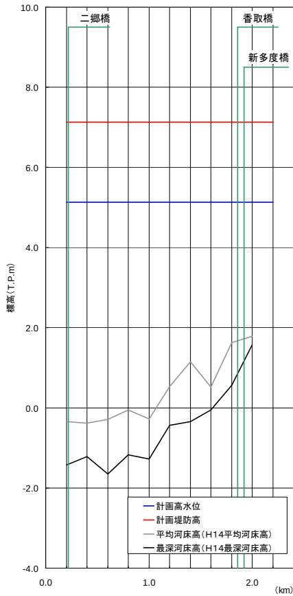
計画諸元表・多度川
