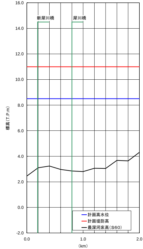
計画諸元表・犀川
