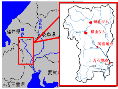
【徳山ダム・横山ダム連携による洪水調節】
