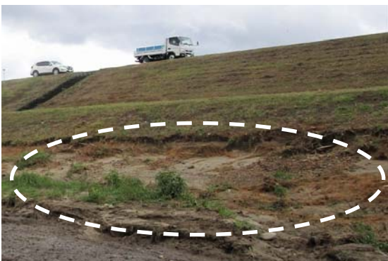
木曾川左岸67.8k 堤防川表の法崩れ状況 (可児市土田地区)
