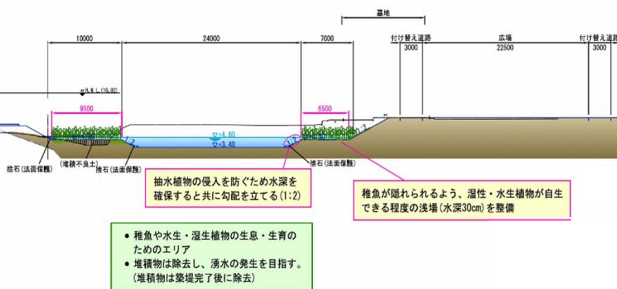
杭瀬川(8.0k付近)再生イメージの断面図
