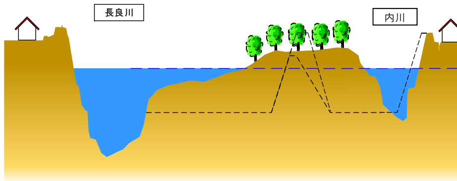
現況河道
