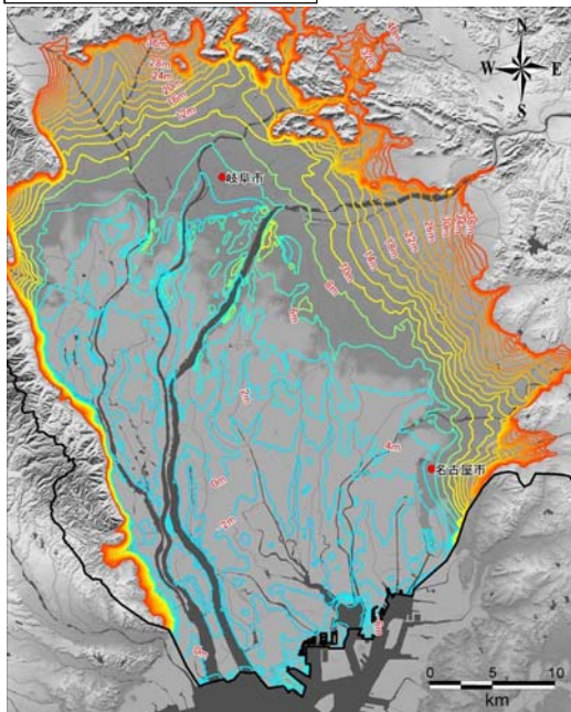
自由地下水面
