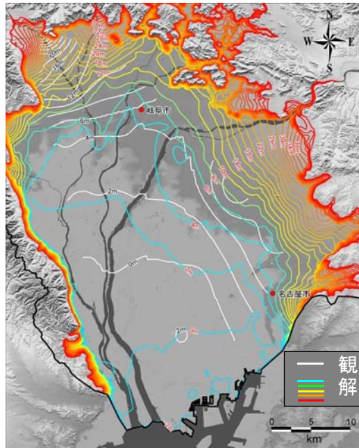
G1礫層の地下水位
