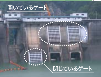
コースターゲート オリフィスゲートを点検する際、ゲートを開けても水を流さないフタの役目を果たします。
