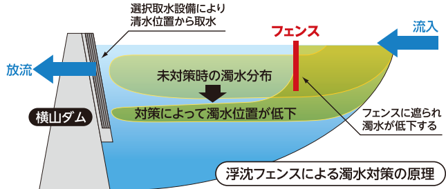
④浮沈フェンス 貯水池の濁りや水温に応じて操作します。選択取水設備と組み合わせることで、下流に流す水の濁りを軽減します。
