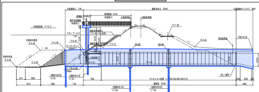
縦断面図
