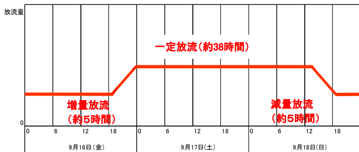
西平ダム地点増量放流のイメージ
