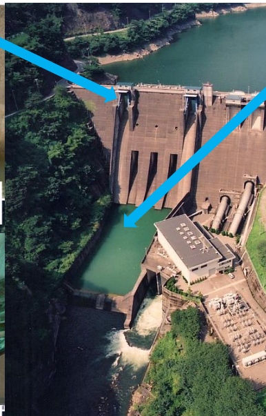
※常用洪水吐ゲート：通常の洪水の際に使用するゲート。 非常用洪水吐ゲート：計画洪水以上の時に使用するゲート。
