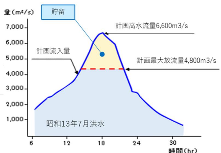
洪水調節図
