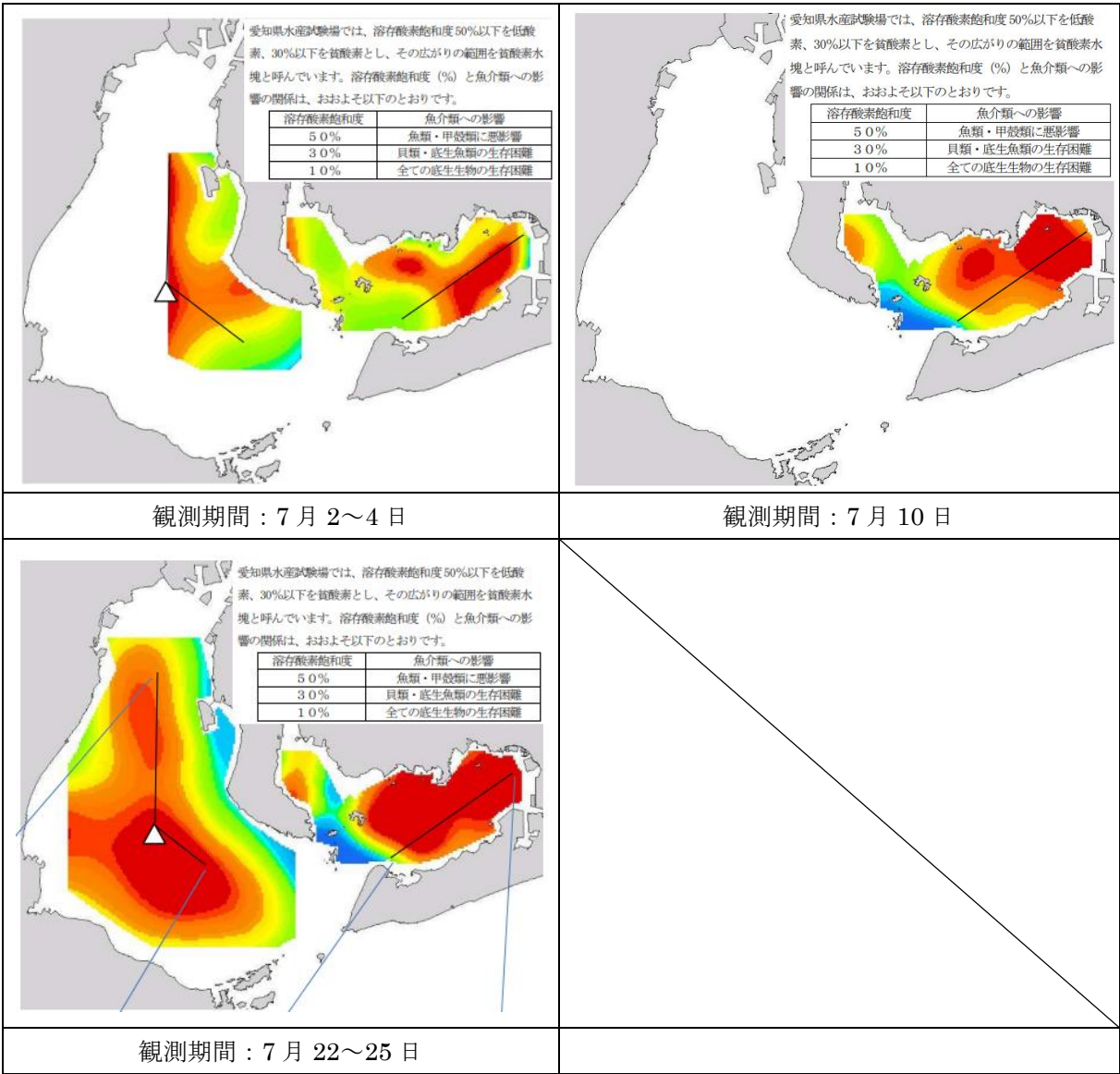
図表の出典：愛知県水産試験場 HP（伊勢・三河湾貧酸素情報） 注）海底付近の DO 分布の中で赤色の部分は、貧酸素水塊となります。
