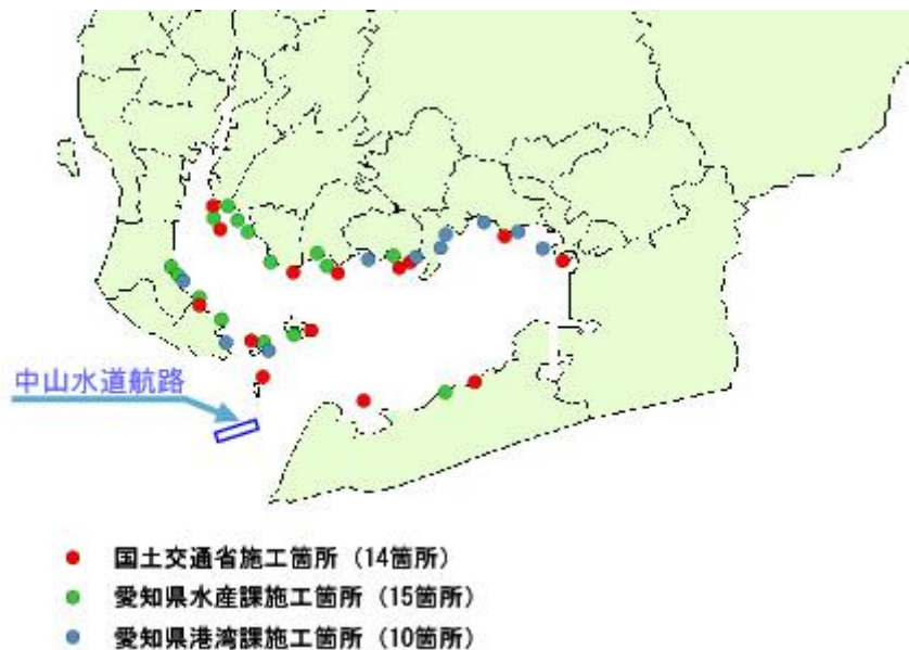
図 15 中山水道航路の浚渫土砂による干潟・浅場造成、覆砂施工箇所
