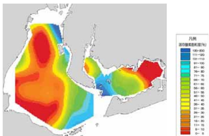
図 17 平成 21 年 9 月の溶存酸素飽和度分布 2 （伊勢湾 9/7,11、三河湾 9/8）
