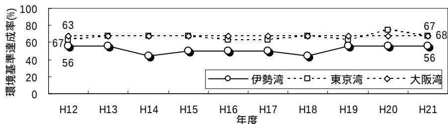
図 10 三大湾の環境基準達成率(COD、水域毎に評価)の経年変化
