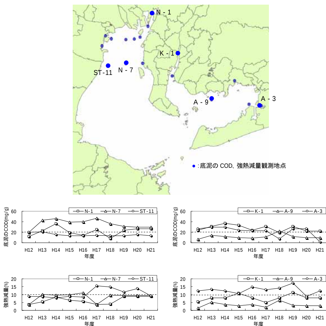
図 18 底泥の COD 及び強熱減量（年平均）の経年変化 （左側：伊勢湾（狭義）、右側：三河湾）
