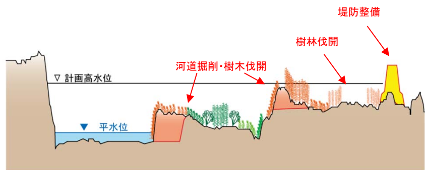
河道掘削の事例・イメージ
