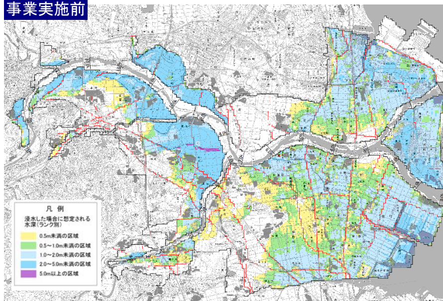
事業実施前の氾濫想定図(河川整備計画目標洪水)
