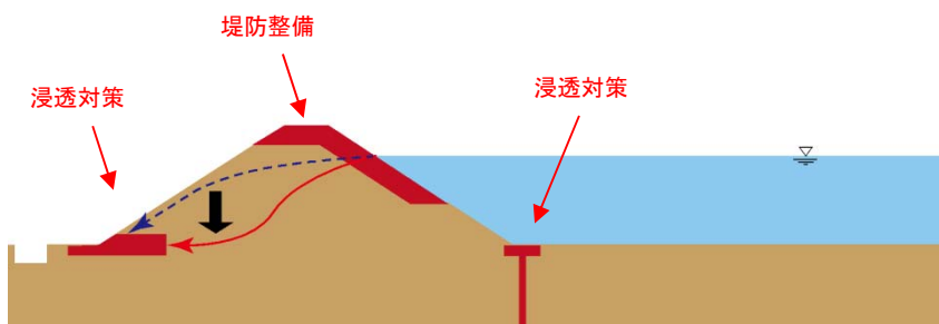
堤防整備・浸透対策のイメージ
