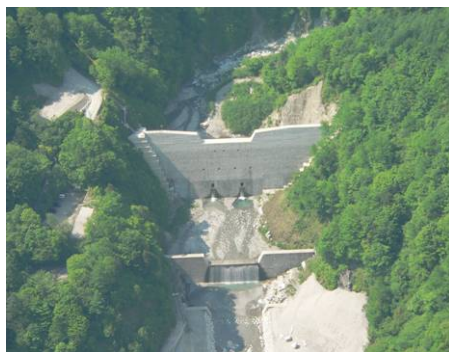
天竜川飯島第6砂防えん堤(不透過型)
